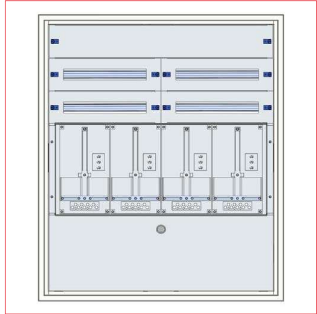
Praxisbeispiel geteilte Frontplatten
